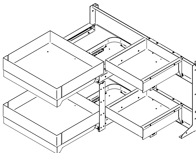
Versione sinistra Left hand version
