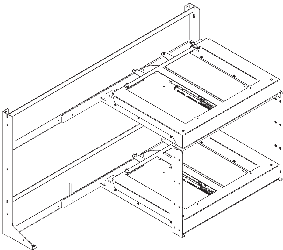
Versione destra Right hand version
